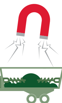
Metal tilbageholdt i en JF-Stoll VM-45 fuldfoderblander monteret med to topmagneter fra Grønning Smede- og Maskinforretning. Foto: SEGES
